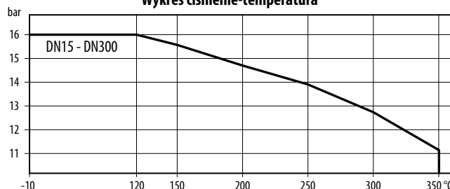
Wykres ciśnienie-temperatura
