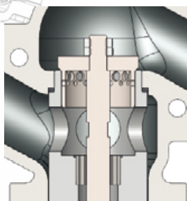
Grzyb perforowany
