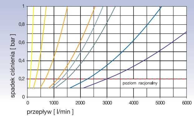
Wykres przepływu dla powietrze (P = 6 bar)
