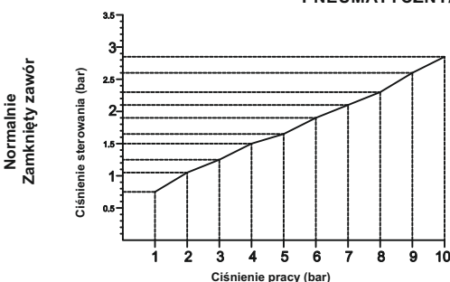
MINIMALNE CIŚNIENIE PRACY - DIAGRAM PNEUMATYCZNY/SPRĘŻYNA ORAZ PILOTY ZASILANE ZEWNĘTRZNIE
