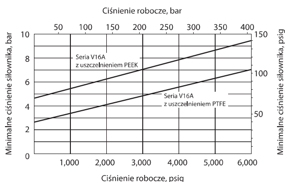
Seria V16A z siłownikiem dwustronnego działania - AD
