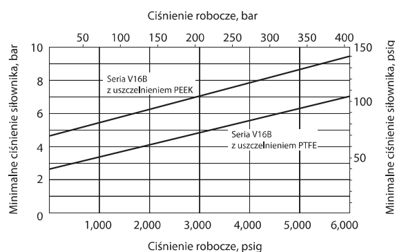
Seria V16B z siłownikiem dwustronnego działania - BD
