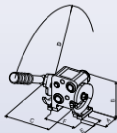
Wymiary, mm
