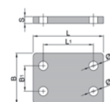
Płyta górna CD PS CP1-7
