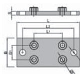
Płyta dolna CD PL CP1-7
