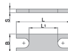
Płytkę pośrednią PB CP1-7
