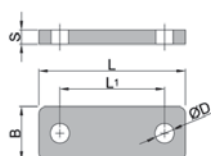
Płytkę górną PS CP1-7
