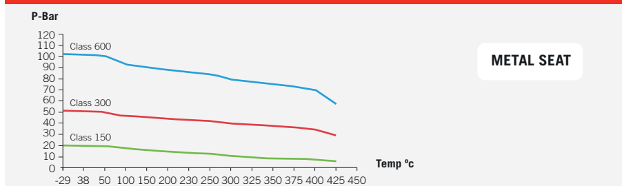
Fig. 2515 (Class 150)
