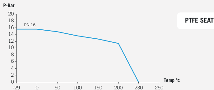
Fig. 916 (PN 16)
