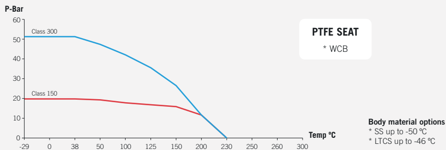
Fig. 515 (Class 150)
