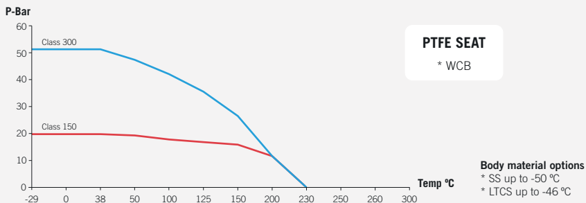
Fig. 1515 (Class 150)
