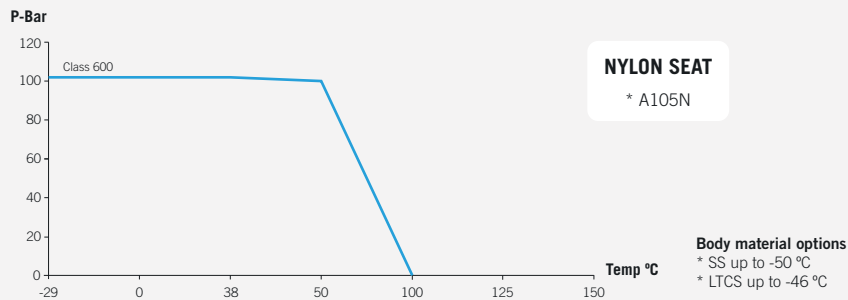
Fig. 560 (Class 600)
