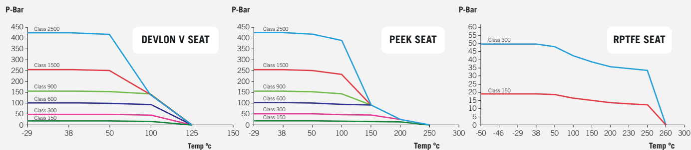
Fig. 6015 (Class 150)
