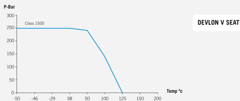
Fig. 81500 (Class 1500)
