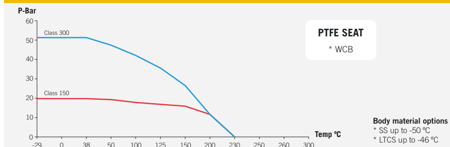
Fig. 715 (Class 150)
