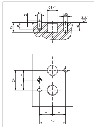
wymiary złącza "NAMUR" zgodnego ze standardem VDI/VDE 3847 (lipiec 2003)
