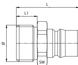
gwint zewnętrzny bez zaworu
