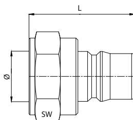
gwint wewnętrzny bez zaworu
