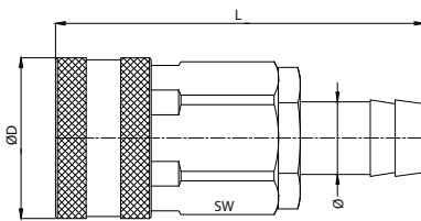
tuleja do węża bez zaworu
