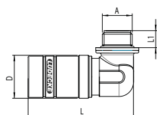
gwint zewnętrzny 90°
