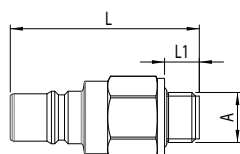
gwint zewnętrzny z zaworem
