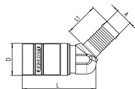
tuleja do węża 45°
