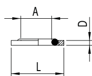
uszczelka FKM
