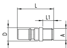
gwint zewnętrzny bez zaworu
