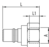
gwint wewnętrzny bez zaworu
