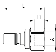
gwint wewnętrzny bez zaworu
