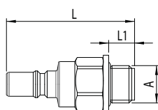
gwint zewnętrzny z zaworem
