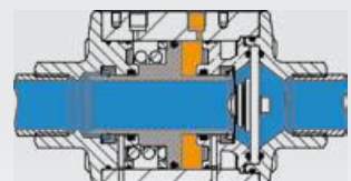
Zawór otwarty
