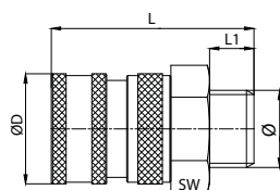
gwint zewnętrzny
