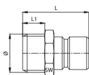
gwint zewnętrzny
