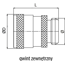
gwint zewnętrzny
