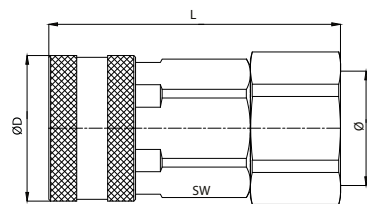
tuleja do węża bez zaworu
