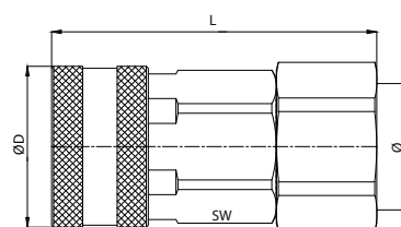
gwint wewnętrzny z zaworem
