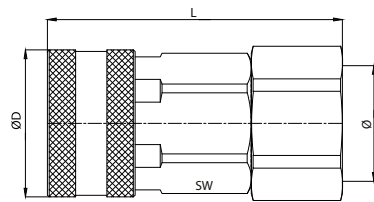
gwint wewnętrzny bez zaworu
