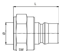
gwint wewnętrzny bez zaworu
