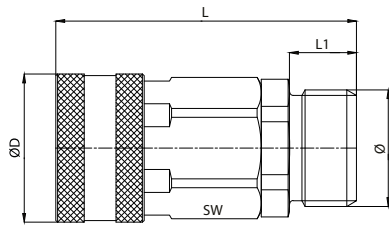
gwint zewnętrzny bez zaworu
