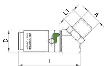
gwint zewnętrzny, 45 stopni
