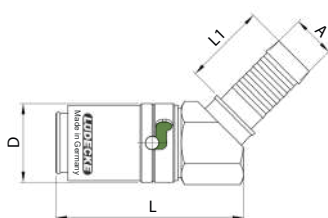
tuleja do węża, 45 stopni
