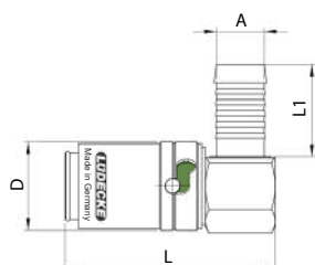
tuleja do węża, 90 stopni
