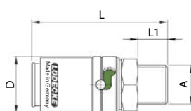
gwint zewnętrzny
