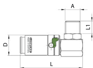
tuleja do węża PUSH-ON, 90 stopni
