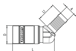
tuleja do węża, 45 stopni
