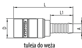
tuleja do węża
