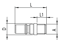
gwint zewnętrzny bez zaworu
