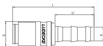
tuleja do węża PUSH-ON
