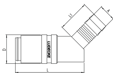
tuleja do węża, 45 stopni
