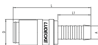
tuleja do węża
