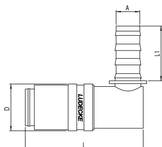
tuleja do węża PUSH-ON, 90 stopni
