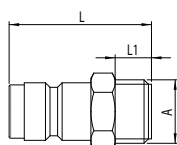
gwint zewnętrzny wewnętrzny stożek 60 stopni bez zaworu
