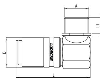
gwint zewnętrzny, 90 stopni
