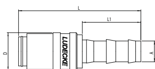
tuleja do węża PUSH-ON
