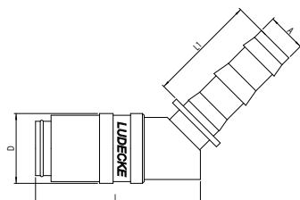
tuleja do węża PUSH-ON, 45 stopni
