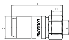
gwint wewnętrzny
