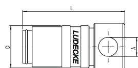
gniazdo do mostka
