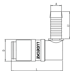
tuleja do węża, 90 stopni
