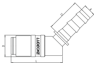
tuleja do węża PUSH-ON, 45 stopni
