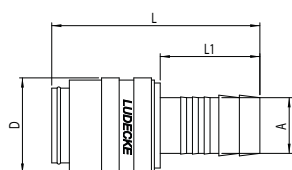
tuleja do węża wersja krótka
