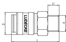
gwint zewnętrzny wersja krótka
