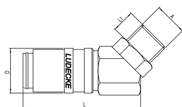
gwint zewnętrzny, 45 stopni
