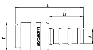
tuleja do węża PUSH-ON wersja krótka
