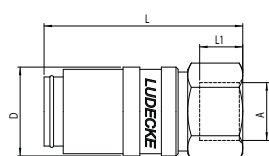
gwint wewnętrzny
