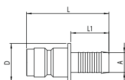
tuleja do węża bez zaworu
