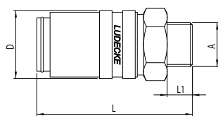
gwint zewnętrzny
