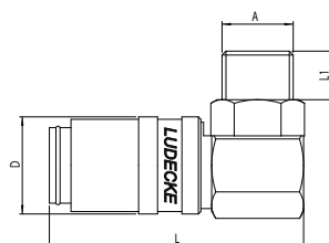
gwint zewnętrzny, 90 stopni
