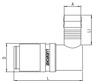
tuleja do węża, 90 stopni
