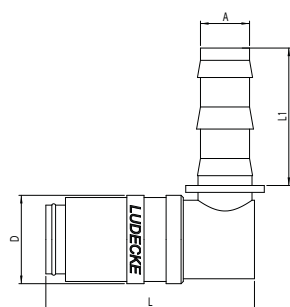
tuleja do węża PUSH-ON, 90 stopni
