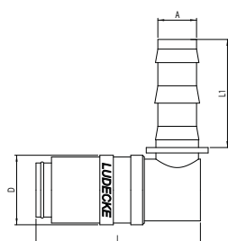
tuleja do węża PUSH-ON, 90 stopni
