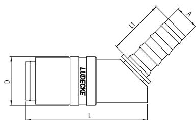
tuleja do węża PUSH-ON, 45 stopni
