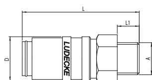
gwint zewnętrzny
