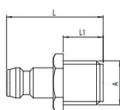
gwint zewnętrzny z zaworem
