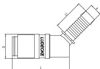
tuleja do węża, 45 stopni
