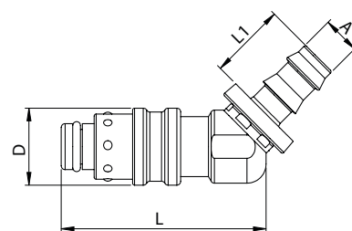
tuleja do węża, 45 stopni PUSH-ON
