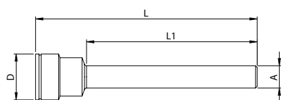
gniazdo przedłużone bez gwintu
