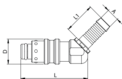
tuleja do węża, 45 stopni
