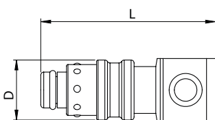
wtyczka do mostków
