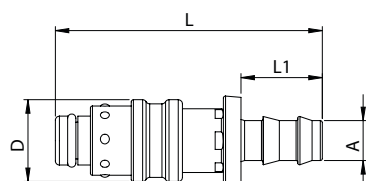
tuleja do węża PUSH-ON
