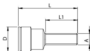
gniazdo przedłużone z gwintem
