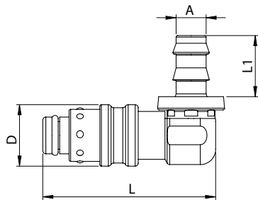
tuleja do węża, 90 stopni PUSH-ON
