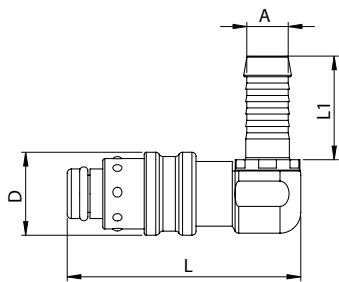
tuleja do węża, 90 stopni
