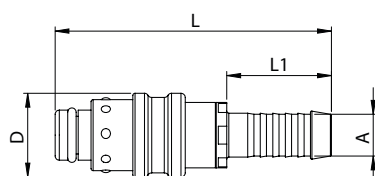
tuleja do węża
