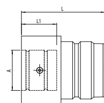
połączenie do rur bez zaworu
