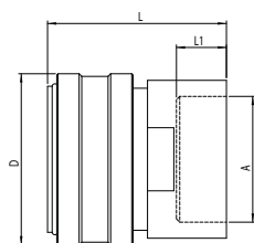
gwint wewnętrzny
