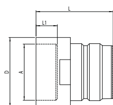
połączenie do rur bez zaworu
