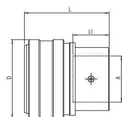
połączenie do rur
