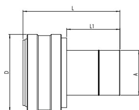
tuleja do węża
